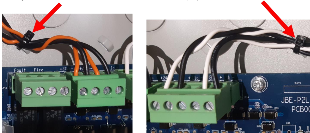
Figura 6: Ilustración de cableado asegurado
