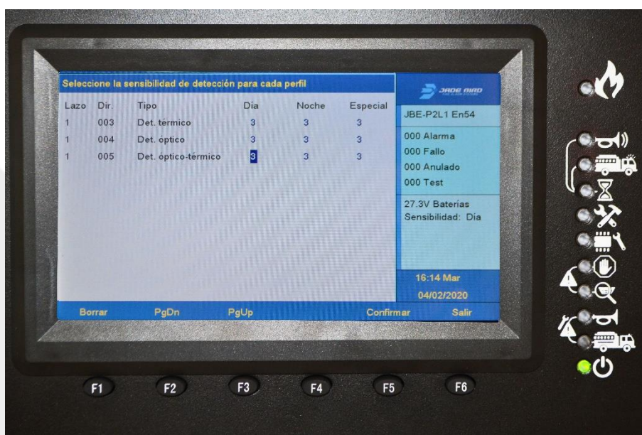
Figura 16: Selección de sensibilidad del detector
