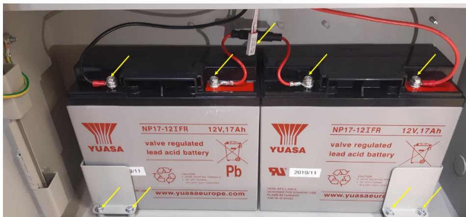
Figura 9: Ubicación de la conexión de la batería para 17 Ah en caja externa
